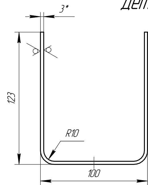
Дет. поз. 1
