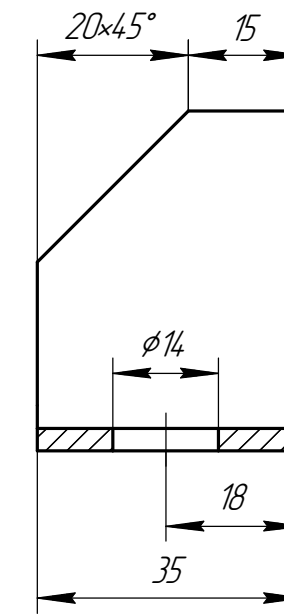
Дет. поз. 3 (1:1)
