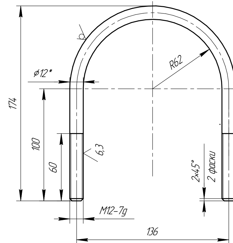
Дет. поз. 5
